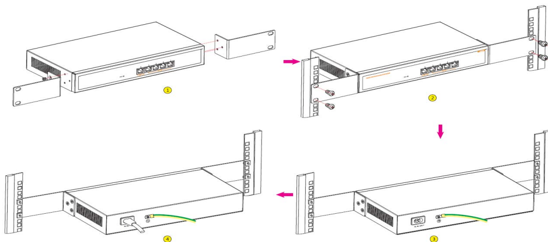
取付手順図
