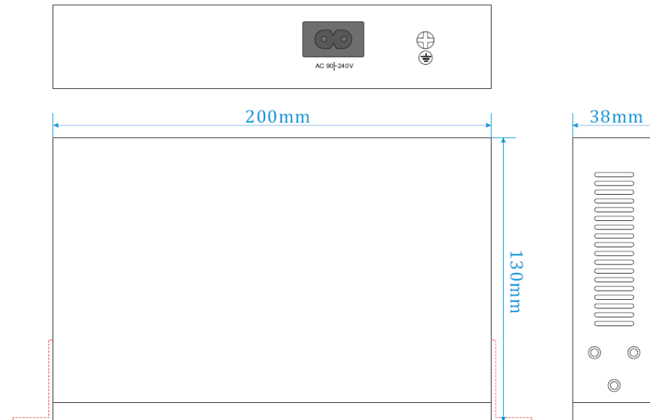
寸法図
